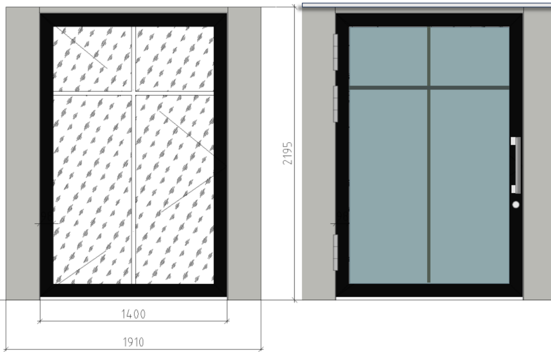
neue Türe / Massskizze FAME AG 6. Feb 2026
